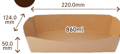
④ CT124×220×H50-860 クラフト(L)
